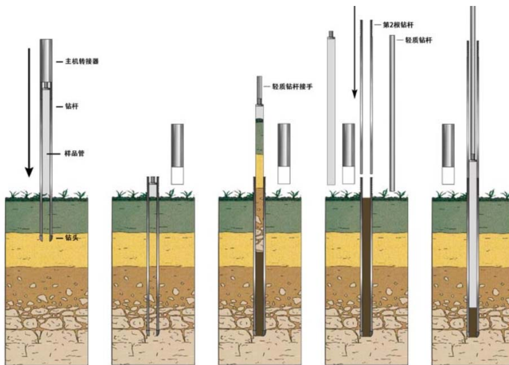
图例 土壤钻探取样示意图
