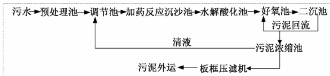
图 2-1 桐乡市濮院恒盛水处理有限公司污水处理工艺流程
