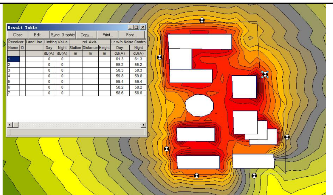
图 7-5 厂界噪声预测点位昼间噪声预测值及等声线图
