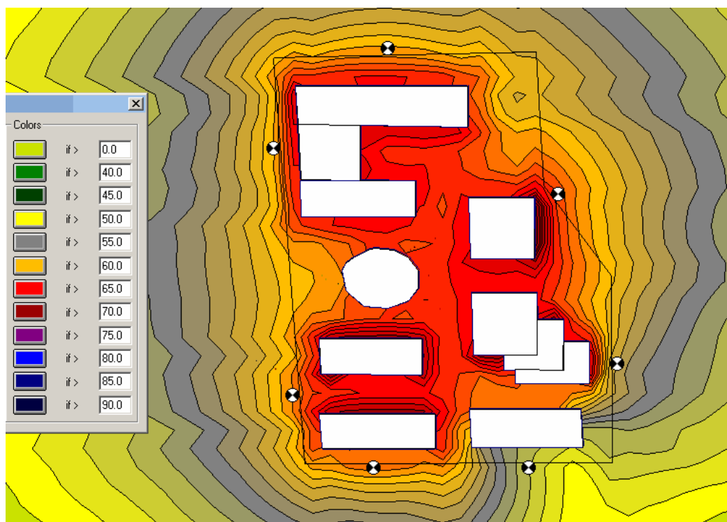
图 7-4 厂界噪声预测点位昼间等声线图
