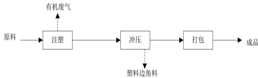
图 5-1 项目生产工艺流程图
