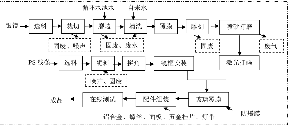
图 5-2 LED 智能灯镜生产流程和产污环节图
