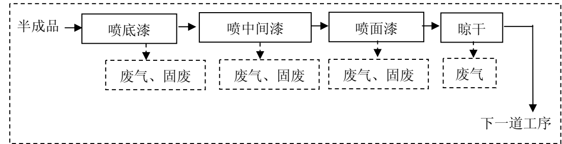
图 5-2 本项目喷漆工艺流程及产污环节
